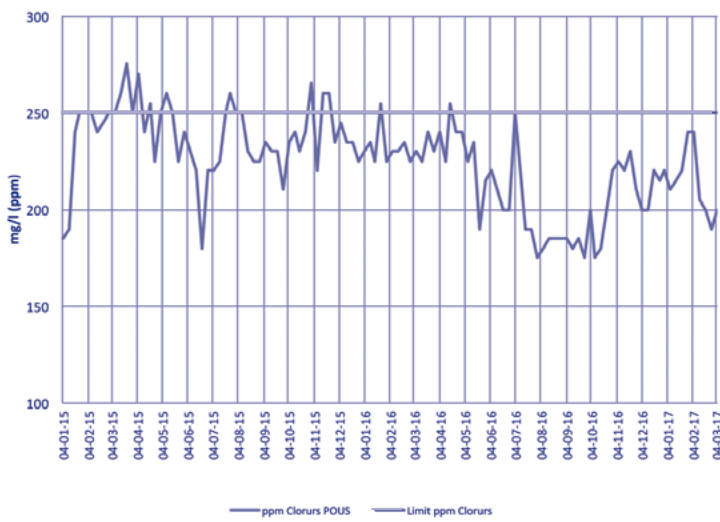
CONCENTRACIÓ DE CLORURS MG/L (PPM) ETAP A XARXA
